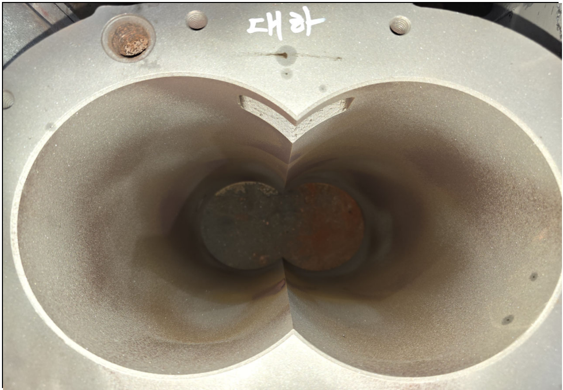
CASING 내경 0.49mm마모, 0.34mm편마모 폐기
